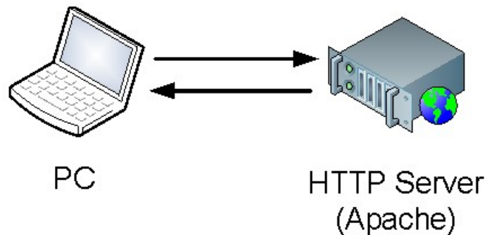
Рис. 1.1. Клієнт-серверна архітектура.
